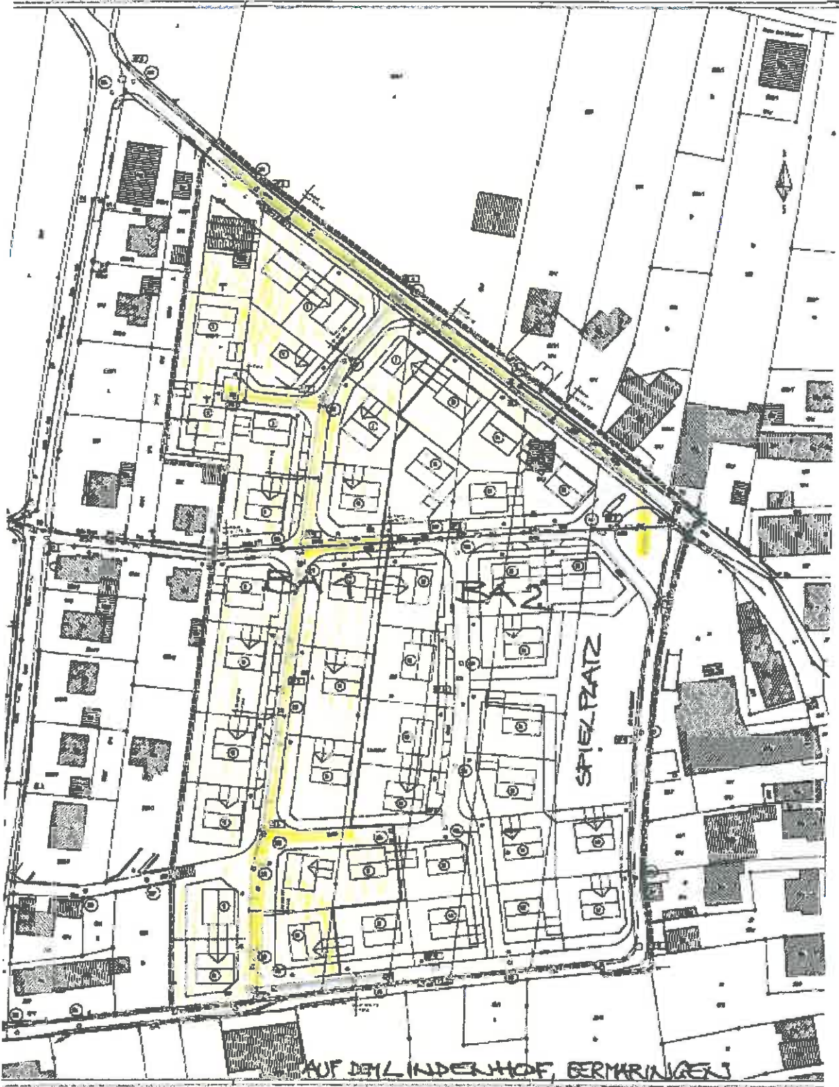
Abb. 1: Bebauungsplan
